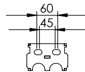
SCHNITT A-A
