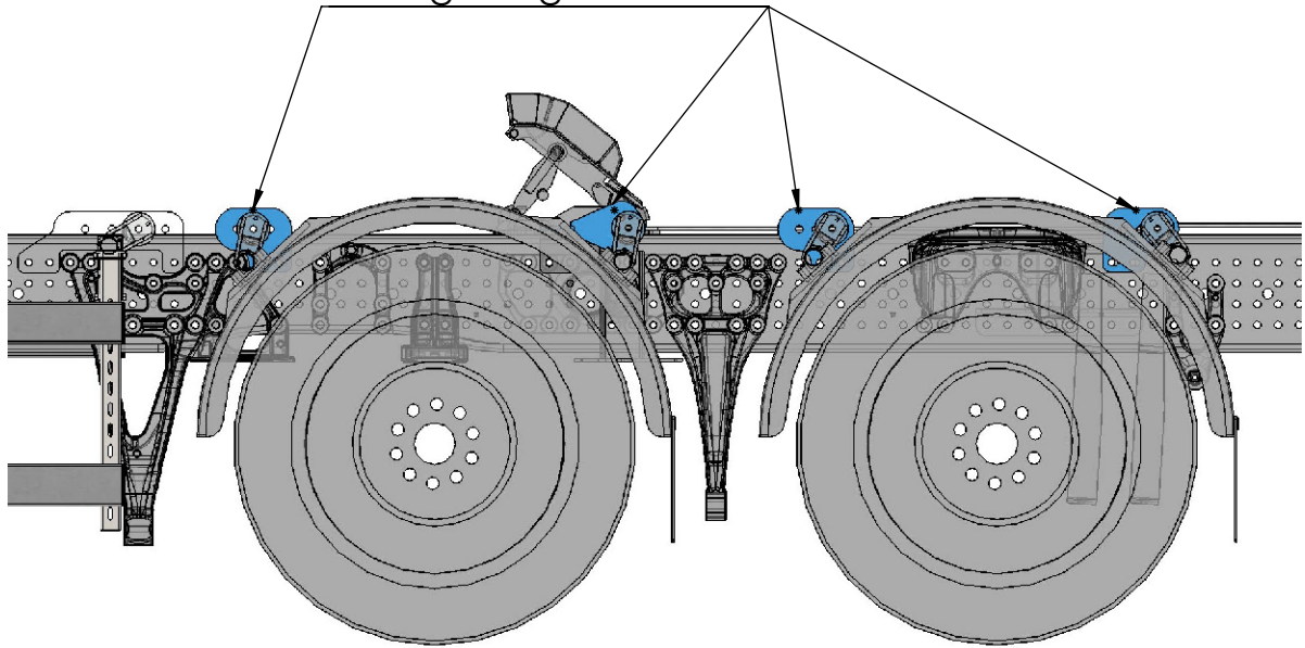
Platten zum Anbau der Kotflügeltragrohre
